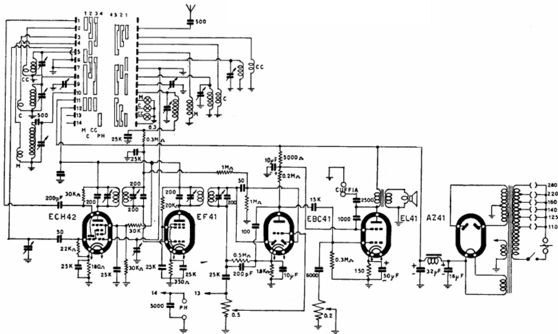
IMCARADIO S. A. - Mod. IF 51. Una gamma onde medie e due gamme onde corte. Commutazione di gamma con tamburo rotante Media frequenza 460 kc. Resa d'uscita 4 watt indistorti.
